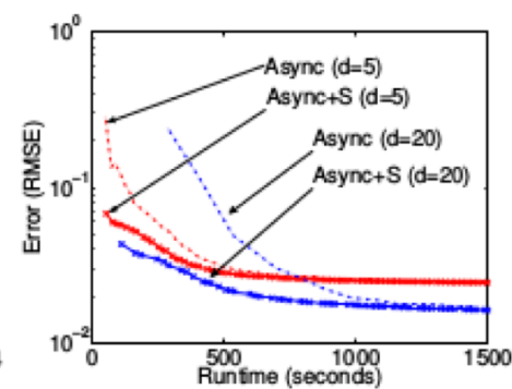
(b) ALS Convergence
