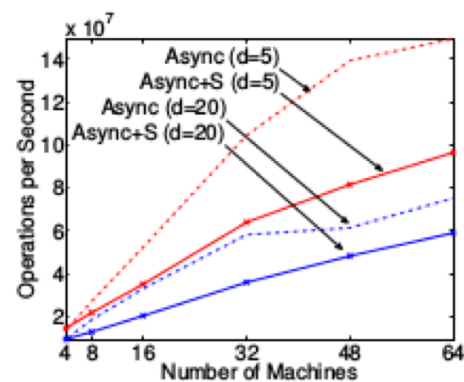
(a) ALS Throughput
